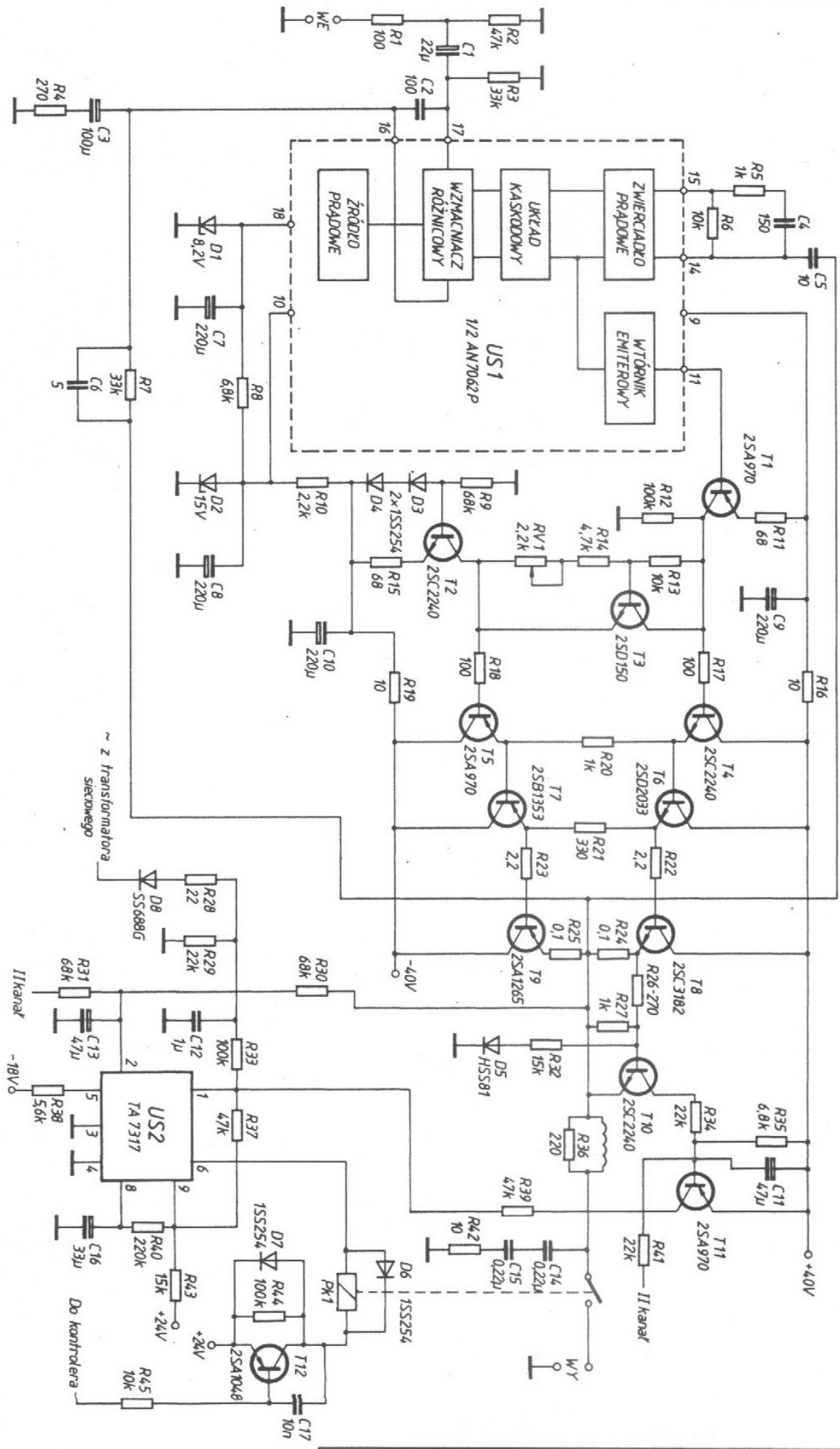
Rys. 2. Schemat stopnia mocy PM66KI ze zmiennami Kena Ishiway
